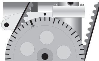
Kąt opóźnienia zapłonu Ignition delay angle Întârziare dinamic
